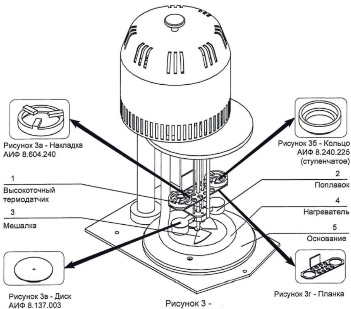
Рисунок 3 – Технологический блок
