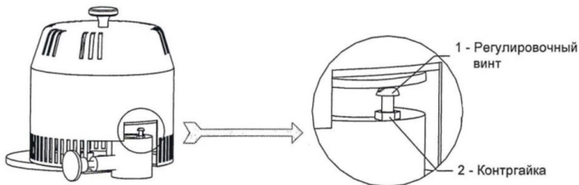
Рисунок 12 – Регулировка высоты подвески
