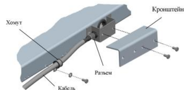
Рис. 5.2 - Подключение кабеля
